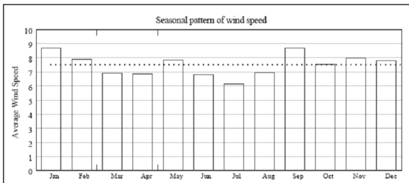
Рисунок 1. Ежемесячные средние скорости ветра на площадке
