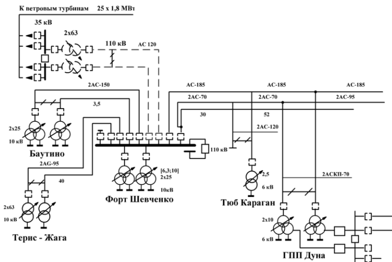
Рисунок 2. Схема подключения ВЭС Форт-Шевченко 45 МВт к электрической сети Мангыстауской области
