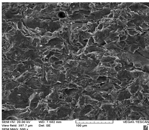
Рисунок 3. СЭМ поверхности, обработанной пескоструйным аппаратом “Air Flow”
