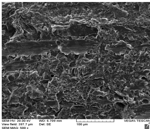
Рисунок 2. СЭМ керамической поверхности, обработанной бором средней абразивности, «Синий», ISO 524
