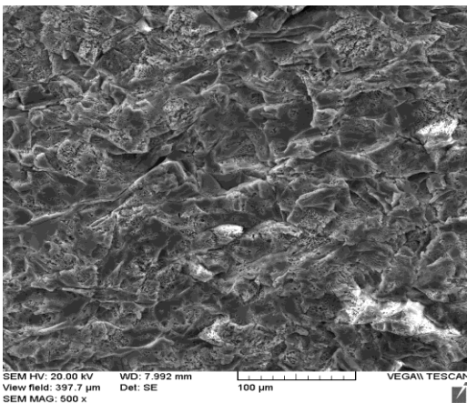
Рисунок 5. СЭМ керамической поверхности, обработанной 9,5 % плавиковой кислотой
