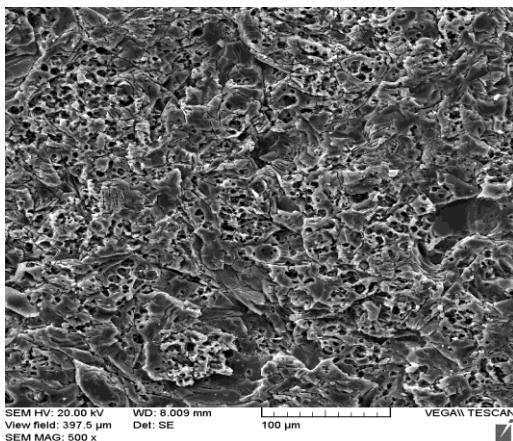
Рисунок 4. СЭМ керамической поверхности, обработанной 4 % плавиковой кислотой
