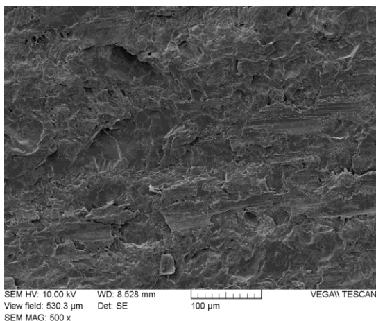
Рисунок 6. СЭМ керамической поверхности, обработанной 37 % ортофосфорной кислотой
