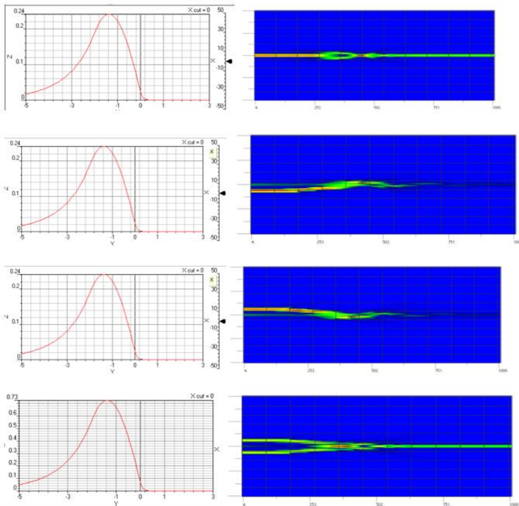
Рисунок 5. Результаты расчета выходной мощности и распределения светового поля в элементе AND при подаче (0,1), (1,0), (1,1)
