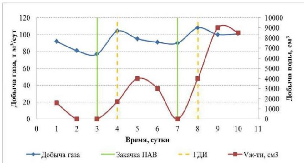
Рисунок 2. Результат испытания ПАВ в 845 скважине
