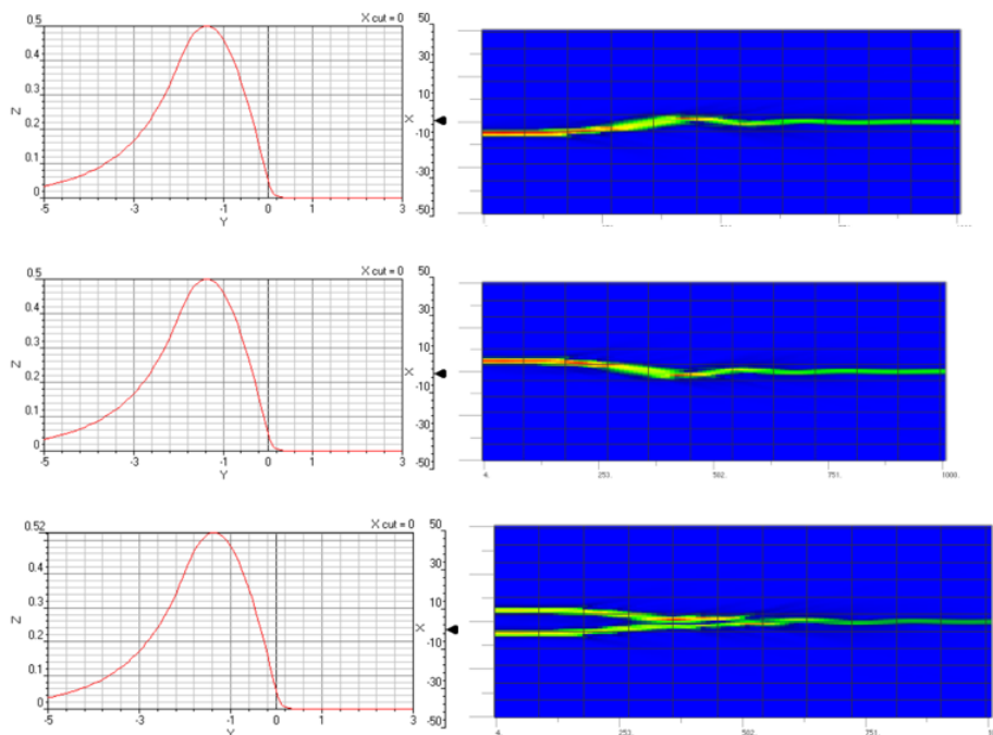
Рисунок 3. Результаты расчета выходной мощности и распределения светового поля в элементе ИЛИ при подаче (0,1), (1,0), (1,1)
