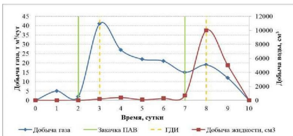
Рисунок 4. Результат испытания ПАВ в 207 скважине
