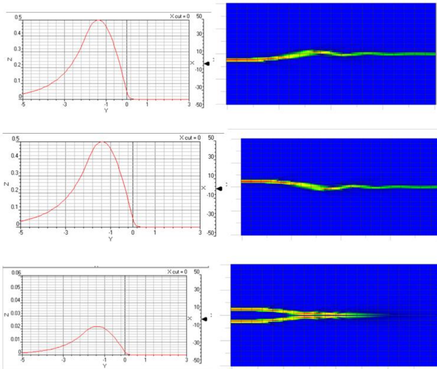
Рисунок 4. Результаты расчета выходной мощности и распределения светового поля в элементе XOR при подаче (0,1), (1,0), (1,1)
