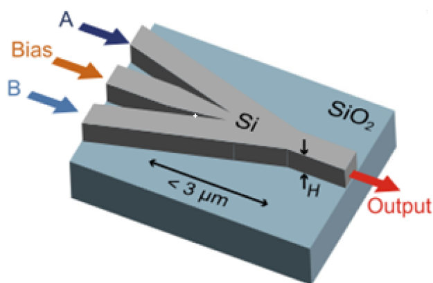
Рисунок 1. Ультракороткий 3-ходовый логический элемент
