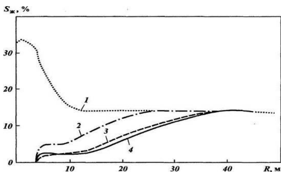
Рисунок 2. Кривые насыщенности коллектора жидкостью в призабойной зоне скважины: 1 – до обработки; 2 – обработка диоксидом углерода; 3 – обработка азотом; 4 – обработка метаном
