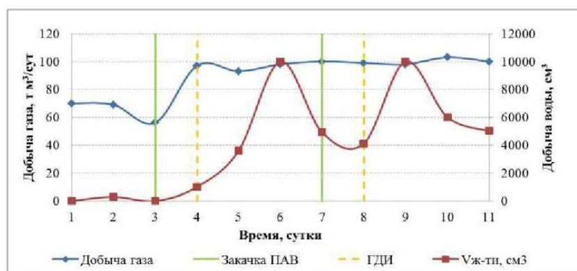
Рисунок 1. Результат испытания ПАВ в 905 скважине
