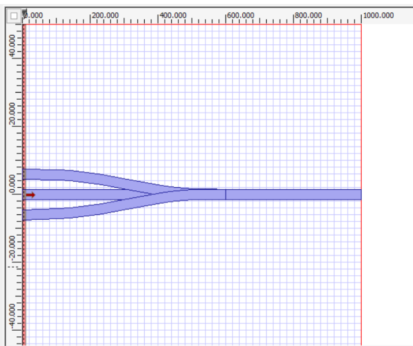
Рисунок 2. Чертеж шаблона логического оптического объединителя
