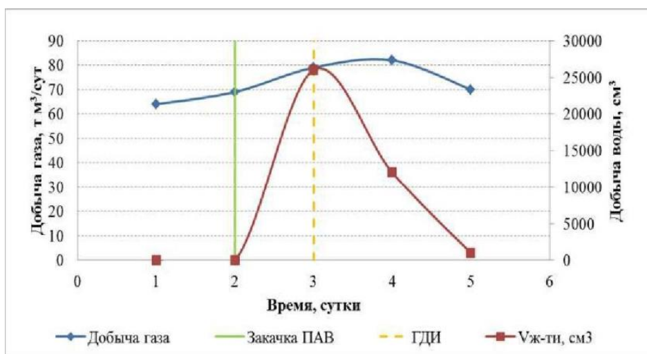
Рисунок 3. Результат испытания ПАВ в 815 скважине
