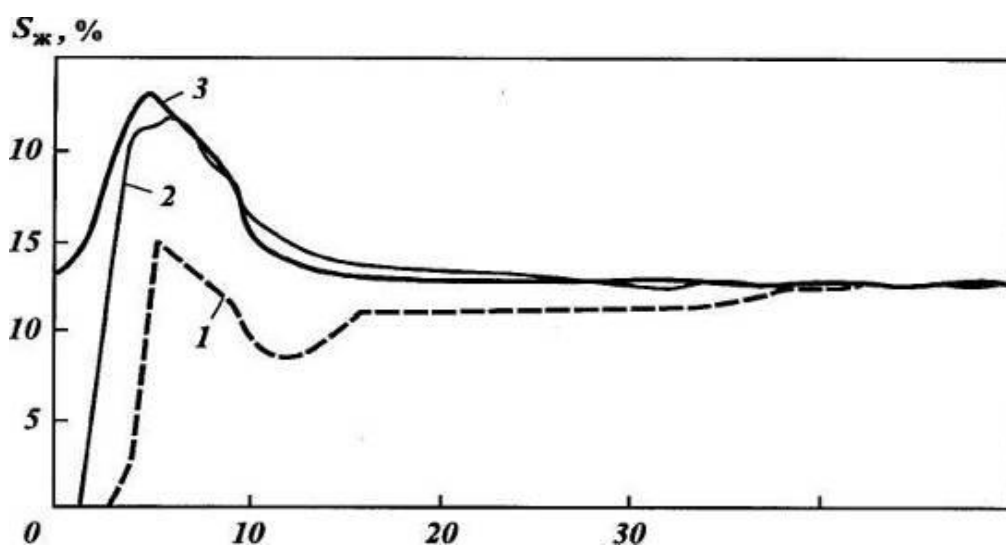
Рисунок 1. Кривые изменения насыщенности коллектора жидкостью в призабойной зоне скважины после обработки сухим газом (1), через 1 месяц (2) и через 4 месяца (3)
