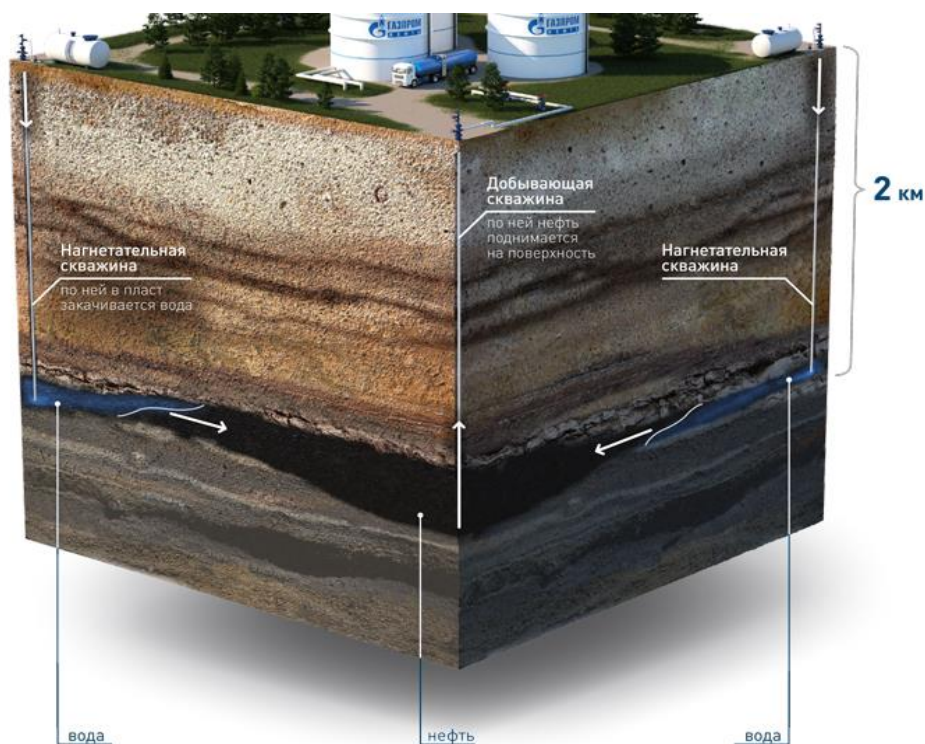
Сурет 1. Қабатқа су айдау процесі
