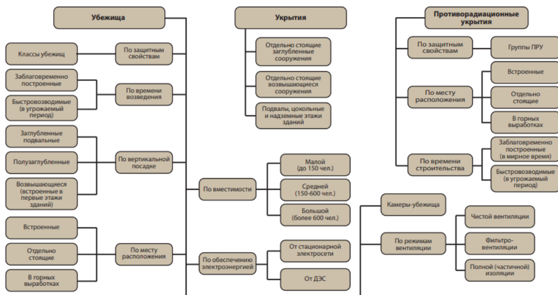
Рисунок 1. Классификация защитных сооружений гражданской обороны [1]
