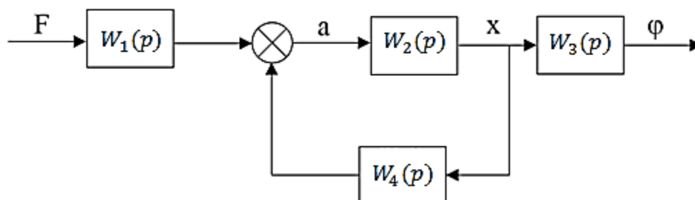
Рисунок 2. Структурная схема системы груз-подвес
