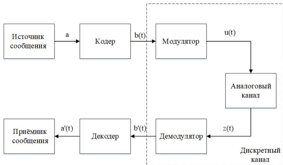
Рисунок 1. Структурная схема системы связи
