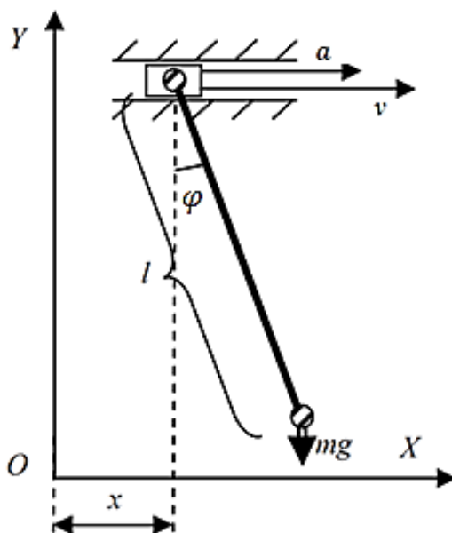
Рисунок 1. Схематичное изображение маятниковой колебательной системы «точка подвеса-груз»
