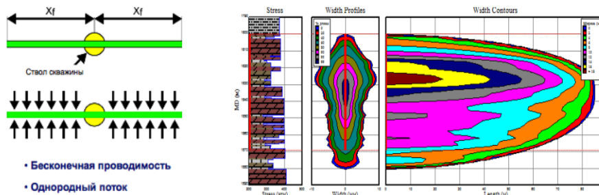
Рисунок 1. Схема трещины ГРП в соответствии с классическим представлением
